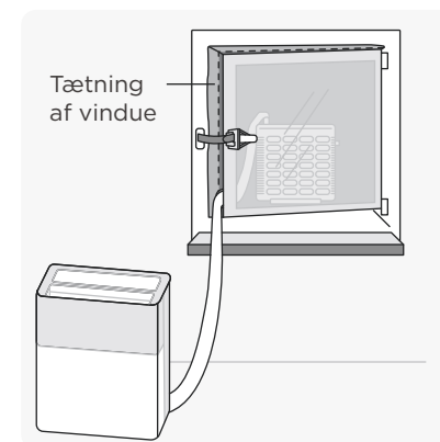
Eksempel på en installeret PortaSplit-vinduestætning.
