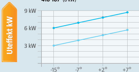
Luft/vatten värmepumpe 416-107 (6 kW)
