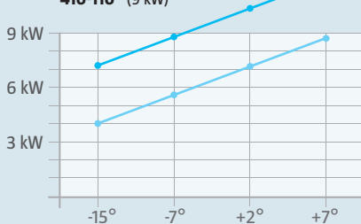
Luft/vatten värmepumpe 416-116 (9 kW)
