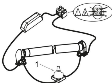
Ferdig ettermontering – LED-lysrørmatur 1 = Forkobling
