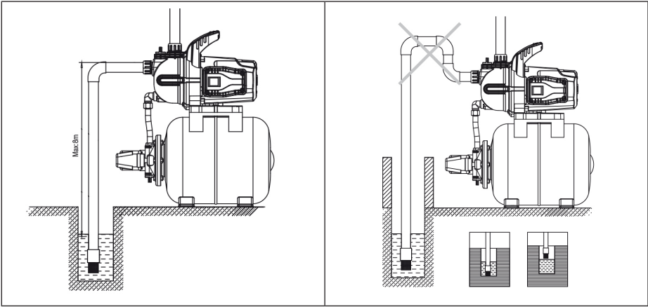
Riktig installasjon
