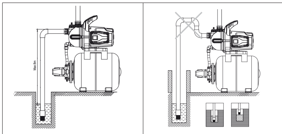
Prawidłowy montaż
