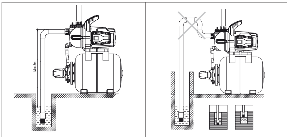
Korrekt installation
